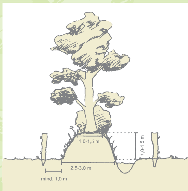
Der typische Aufbau einer Wallhecke.
